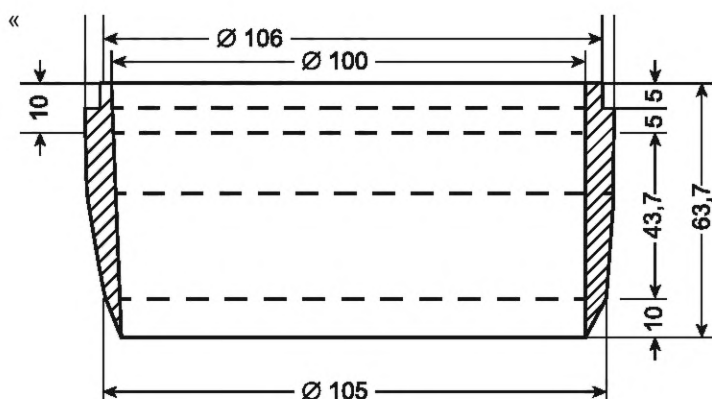
Рисунок 1 — Схема режущего кольца.
